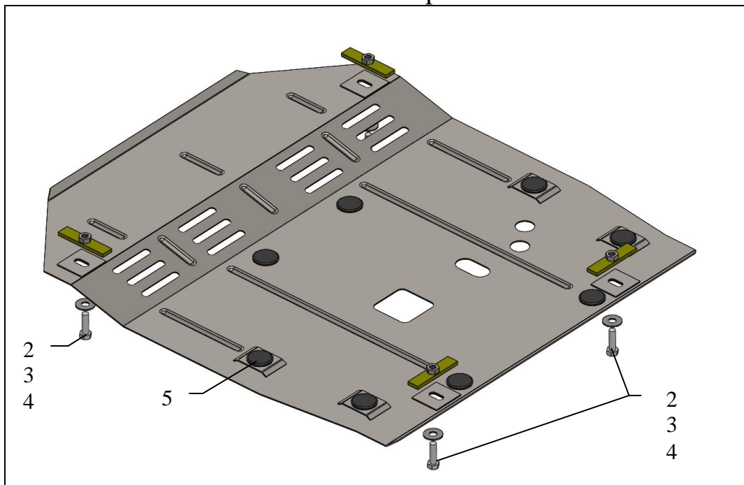
Схема сборки
