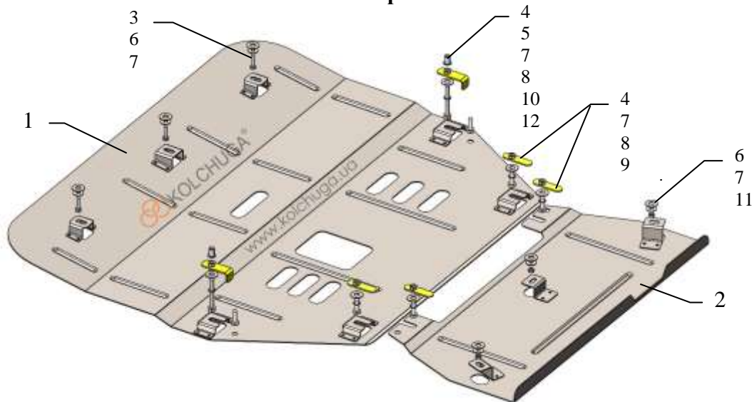
Схема сборки.
